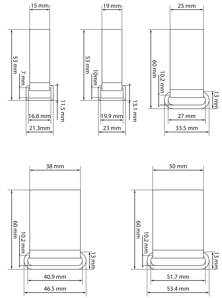
DIMENSIONEN (MM) DER RIEMEN-SCHLAUFEN IN STANDARDAUSFÜHRUNG
