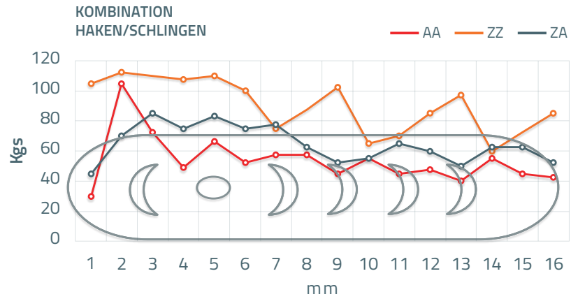
ABREISSFESTIGKEITSTEST HAKEN/SCHLINGEN VERSUS KONTAKTZONE
