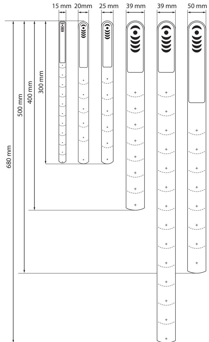
DIMENSIONEN (MM) DER GURTBÄNDER IN STANDARDAUSFÜHRUNG
